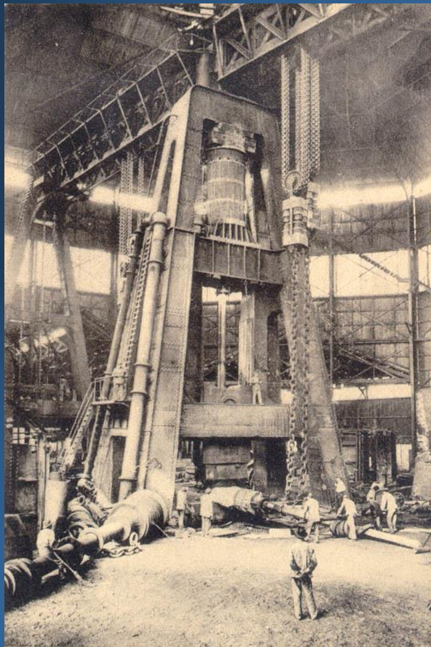
TERNI - Acciaierie Maglio di 108 Tonnellate (il più grande del mondo)
