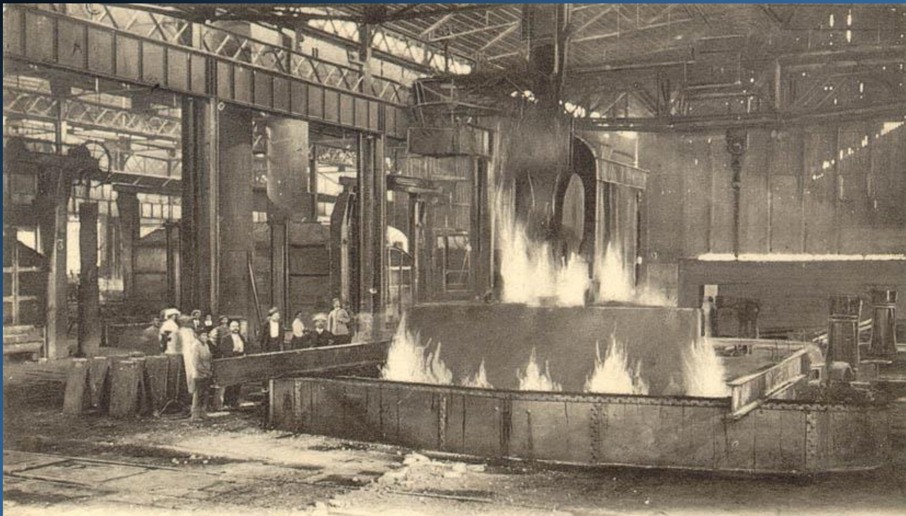
Acciaierie di Terni - Tempera all'olio di una corazza da 28 tonnellate
