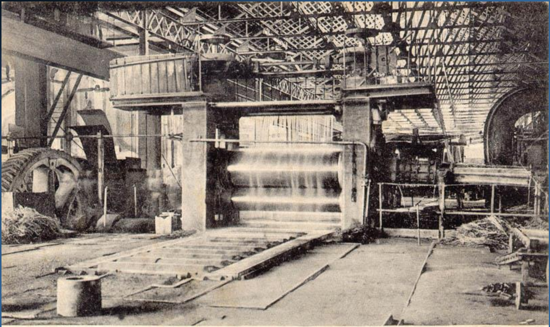
Acciaierie di Terni - Laminatoio per corazze da 40 tonnellate
