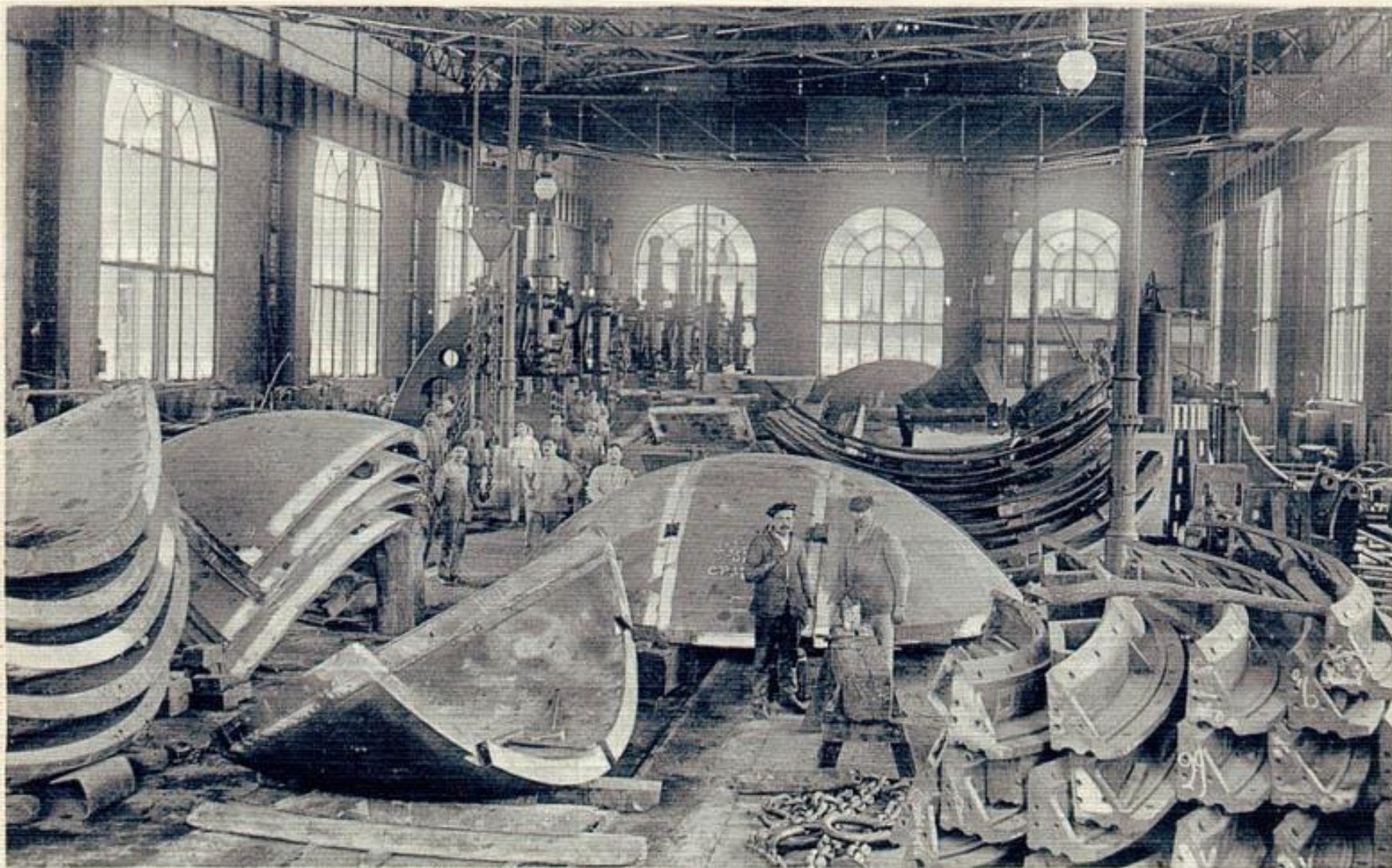
TERNI (Acciaierie) - Officina finimento cupole corazzate
