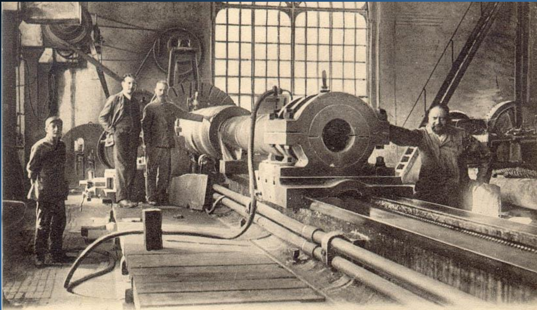
Acciaierie di Terni - Officina torneria cannoni (parte di campata sud-ovest)
