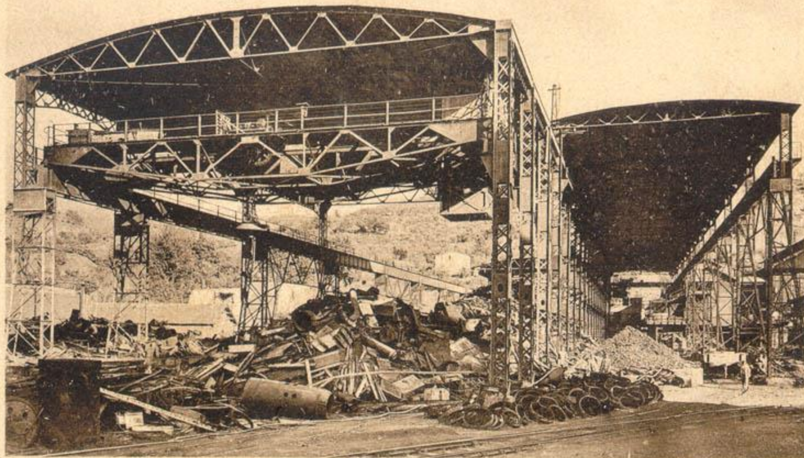
ACCIAIERIE DI TERNI Grue equipaggiata da motore chiuso C.G.E. da 80 HP
